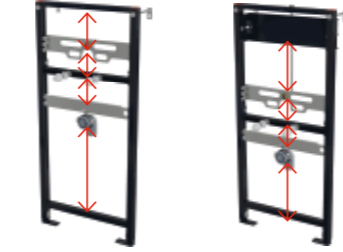
A107/1120 Монтажная рама для писсуара A107S/1120 Монтажная рама для писсуара и сенсорного устройства
