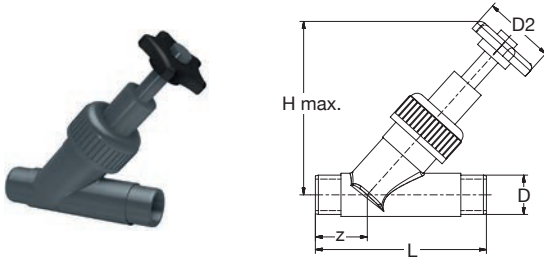
BR PVC-U Ventil Schrägsitz Runddichtring-EPDM grau BR PVC-U Valve angle seat O-Ring-gasket-EPDM grey
