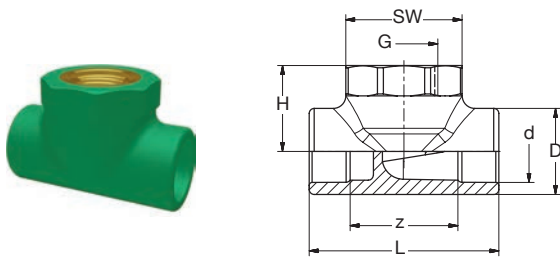
BR PP-RCT-LFB Ventil Geradsitz Unterteil IG-zyl grün
