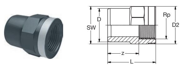
BR PVC-U Ü-Reduktion IG-zyl grau
