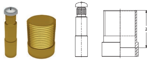
BR Ventil Geradsitz UP Verlängerungsset 25mm
