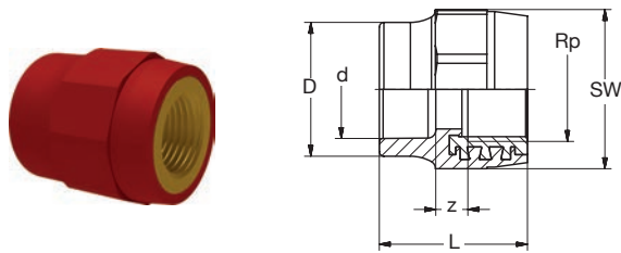
BR PP-CFR- Ms/LFB Übergang IG-zyl rot
