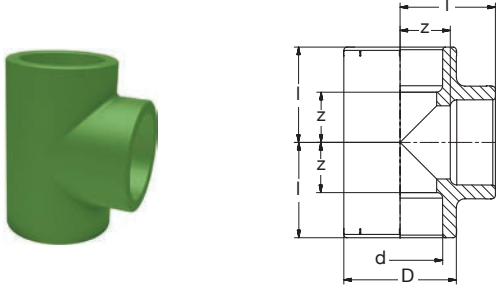
BR PP-R T-Stück 90° grün BR PP-R Tee 90° green
