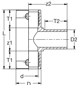
BR PE100 E-T-Stück 90° red mit Schweißstutzen SDR11 schwarz NEU BR PE100 E-Tee 90° red. with spigot SDR11 black NEW
