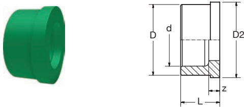
BR PP-RCT Verschraubung Einlegeteil grün BR PP-RCT Union Insert-part green
