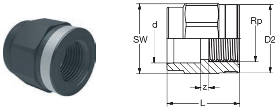
BR PVC-U Übergang IG-zyl grau
