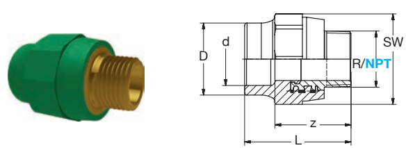
BR PP-RCT-RG/LFB Übergang AG-keg grün
