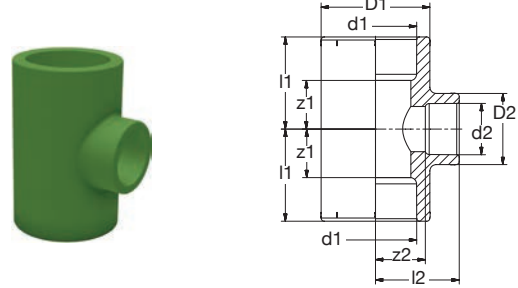
BR PP-R T-Stück 90° red grün BR PP-R Tee 90° red green
