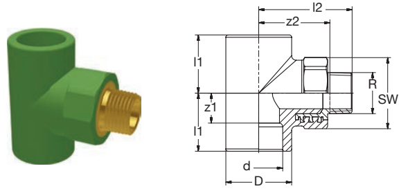
BR PP-R-RG/LFB Ü-T-Stück 90° AG-keg grün
