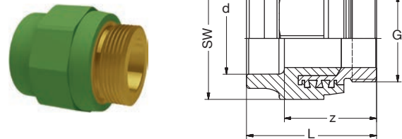
BR PP-R- RG/LFB Verschraubung Schraubteil flachdichtend grün BR PP-R- Bronze/LFB Union Srew-part flat-sealing green
