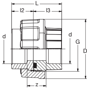
BR PP-R Verschraubung Runddichtring-EPDM 20°C/ 1,0MPa grün BR PP-R Union O-Ring-gasket-EPDM 20°C/ 1.0MPa green
