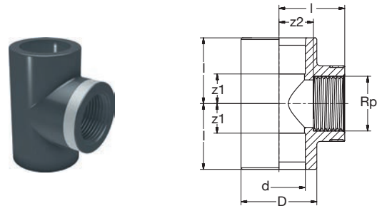
BR PVC-U Ü-T-Stück 90° IG-zyl grau
