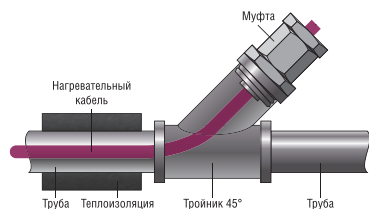
Схема 1. Монтаж муфты в тройник 45°
