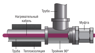
Схема 2. Монтаж муфты в тройник 90°
