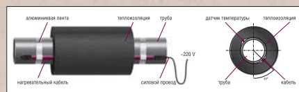
Монтаж кабеля на трубу
