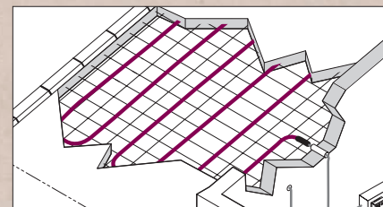
Размещение кабеля на подъездных путях
