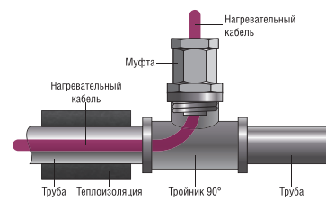
Схема 2. Монтаж муфты в тройник 90°
