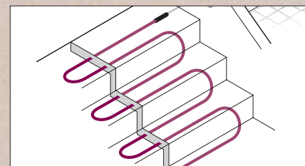
Размещение кабеля на лестнице
